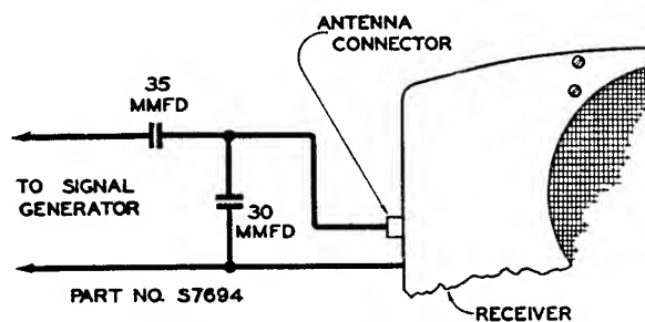
Fig. 3. Dummy Antenna
